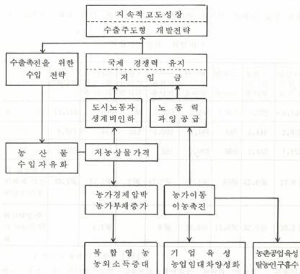
〈개방농정의 기본구조〉 46)
